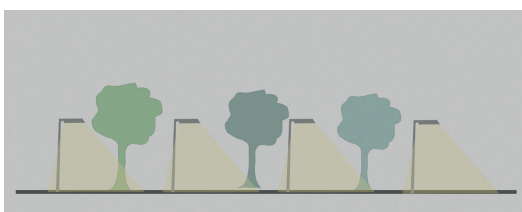
Abbildung 5.5 Kombinierte Wirkung von abgeschirmten Leuchten und kurzen Masten zur Begrenzung der störenden Lichtausbreitung in angrenzende Räume (Engl.: „light trespass“). Erstes Bild – nicht abgeschirmte Leuchten, zweites Bild – abgeschirmte Leuchten. Das dritte Bild zeigt abgeschirmte Leuchten auf kurzen Masten, die die ungewollte Lichtausbreitung verhindern und somit benachbarte Bereiche dunkel halten (© H. LIMPENS).
