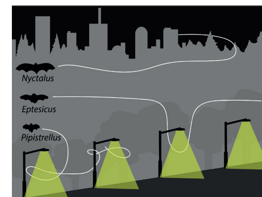
Abbildung 2.7 Schematische Darstellung des Zusammenhangs von Körpergröße und Flügelform und der typischen Nutzung des Luftraumes um eine Reihe von Straßenlaternen durch Fledermäuse verschiedener Gattungen. Die kleinsten Fledermäuse, wie z.B. P. pipistrellus , fliegen normalerweise nur um jeweils eine oder wenige Laternen und halten sich auch eine bestimmte Zeit im jeweiligen Lichtkegel auf. Fledermäuse der Gattung Eptesicus patrouillieren in der Regel entlang der gesamten Laternenreihe und unternehmen kurze Sturzflüge in den Lichtkegel, um Insekten, normalerweise Nachtfalter, zu jagen. Fledermäuse der Gattungen Nyctalus und Vespertilio sind selten im Lichtkegel kleiner Straßenlaternen, aber gelegentlich in solchen größerer Lichtquellen wie Flutlichtern zu sehen (© J. EKLÖF).
