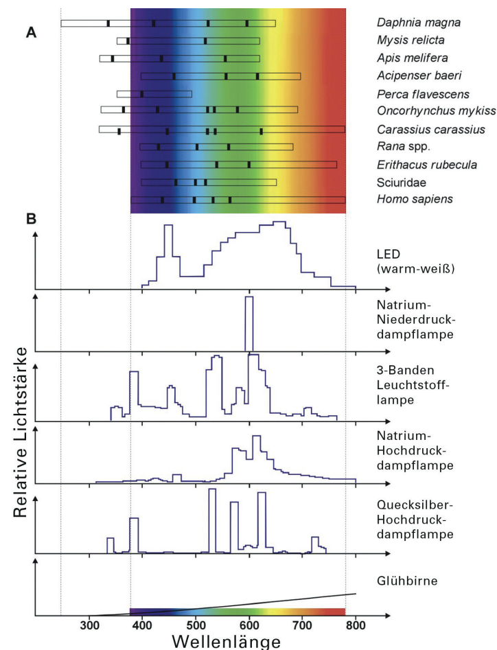
Abbildung 1.6 (A) Die Lichtempfindlichkeit des Sehsinns verschiedener Tierarten im Spektrum des für den Menschen sichtbaren Lichts. Die gestrichelten vertikalen Linien begrenzen den Wellenlängenbereich, den die aufgeführten Arten wahrnehmen können. Die schwarzen Markierungen in den Balken zeigen den Wellenlängenbereich der höchsten Empfindlichkeit der Sehpigmente der kleinen Krebstiere Daphnia magna und Mysis relicta , des Insektes Apis mellifera (Honigbiene) und der Fische Acipenser baeri (Stör), Perca flavescens (Barsch), Onchorhynchus mykiss (Forelle) und Carassius carassius (Karpfen) sowie von Amphibien Rana spp. (Frösche), des Vogels Erithacus rubecula (Rotkehlchen) und der Säugetiere Sciuridae (Eichhörnchen) und Homo sapiens (Mensch). Abbildung (B) zeigt die Wellenlängen des Lichts, das von einer Reihe künstlicher Lichtquellen emittiert wird. Einige Lampen strahlen Licht im UV-Bereich ab. Die Breite des emittierten Spektrums variiert je nach Lampentyp erheblich © PERKIN et al. (2011).
